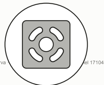
SAPATA / FLANGE placa 200×200mm · chapa 3/8" furos oblongos em curva — nivelamento
