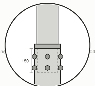
EMENDA MÓVEL encaixe de 150mm com luva de emenda 6 parafusos sextavados — espaçamento 120°
