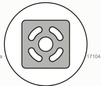
SAPATA / FLANGE placa 200×200mm · chapa 3/8" furos oblongos em curva — nivelamento
