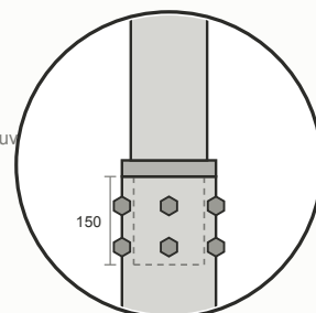
EMENDA MÓVEL encaixe de 150mm com luva de emenda 6 parafusos sextavados — espaçamento 120°
