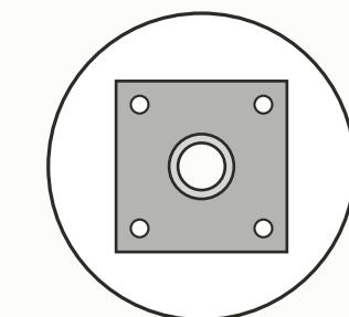
SAPATA / FLANGE placa 200×200mm · chapa 3/8" 4 furos para chumbador
