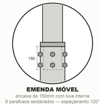
EMENDA MÓVEL encaixe de 150mm com luva interna 6 parafusos sextavados — espaçamento 120°
