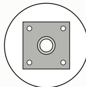
SAPATA / FLANGE placa 200x200mm · chapa 3/8" 4 furos para chumbador
