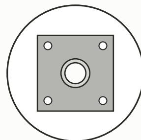
SAPATA / FLANGE placa 200×200mm · chapa 3/8" 4 furos para chumbador
