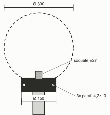
DETALHE — BOCA & GLOBO globo PVC 15x30 incluso · lâmpada não inclusa
