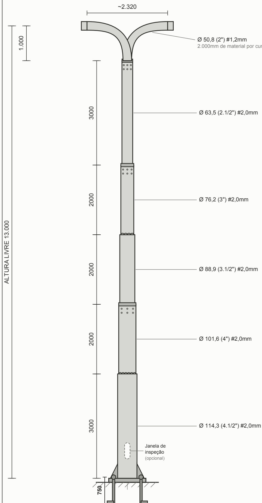
VISTA LATERAL — FLANGEADO medidas em mm
