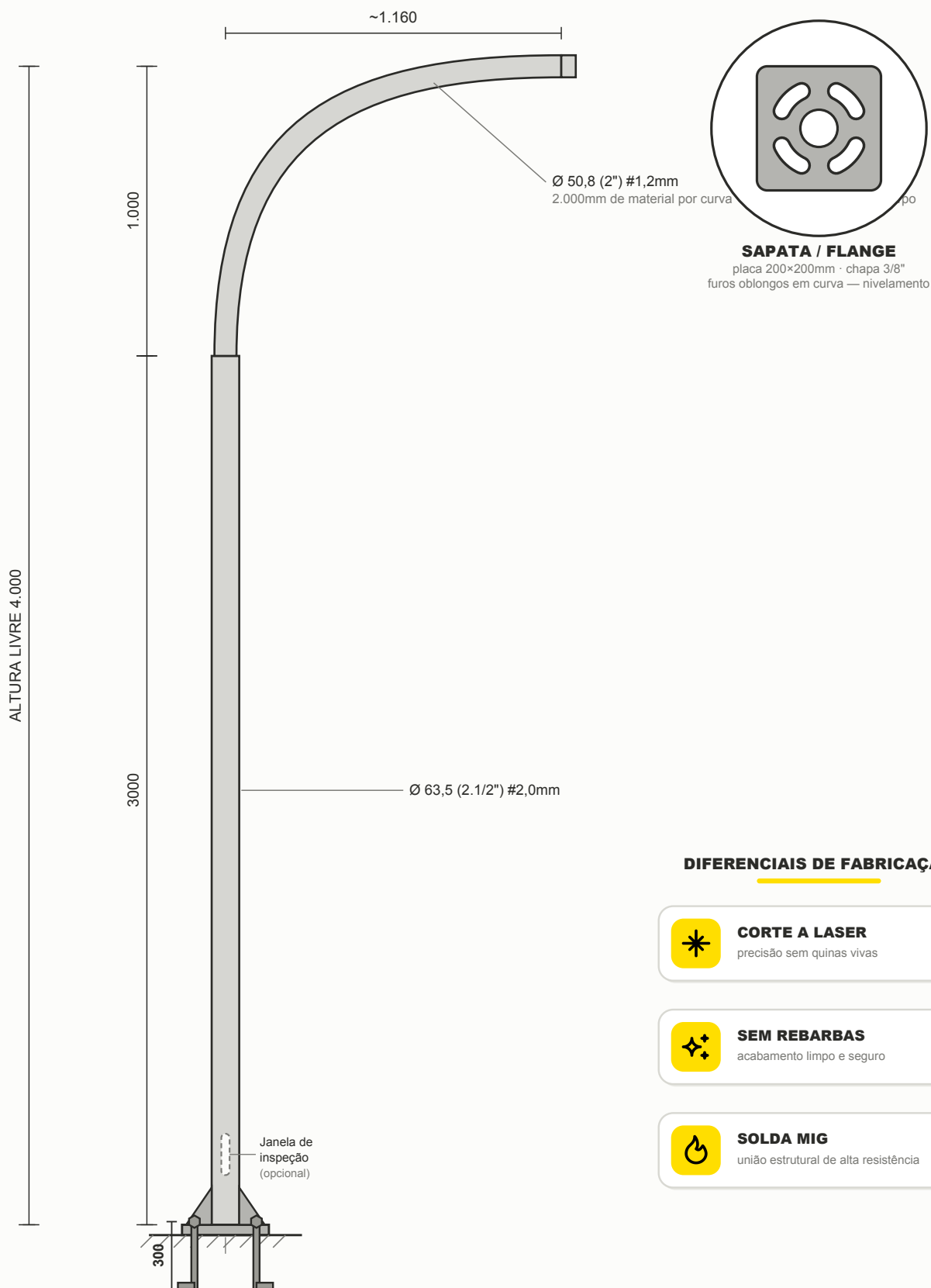
VISTA LATERAL — FLANGEADO medidas em mm
