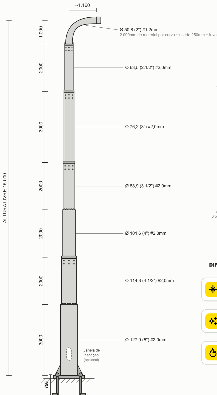
VISTA LATERAL — FLANGEADO medidas em mm
