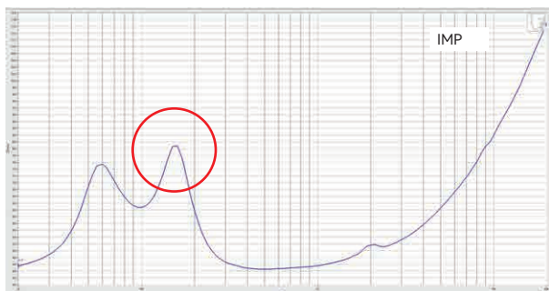
倒相管设计
