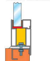
Telaio con controtelaio
