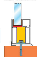
Telaio a tassellare
