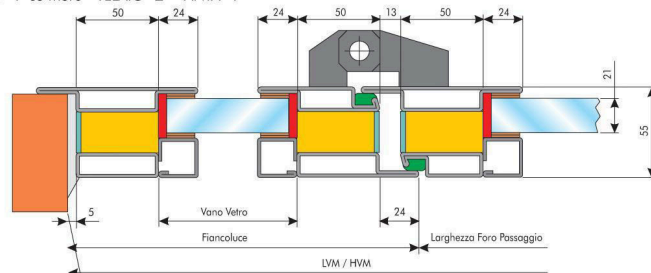
Telaio a T
