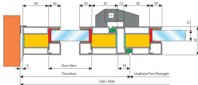
TELAIO "T" su muro - TELAIIO "Z" - ANTA "T"
