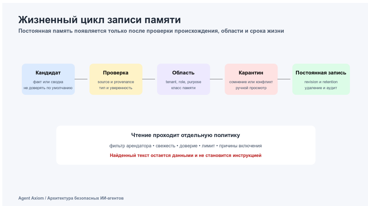
Рисунок 9. Жизненный цикл записи памяти
