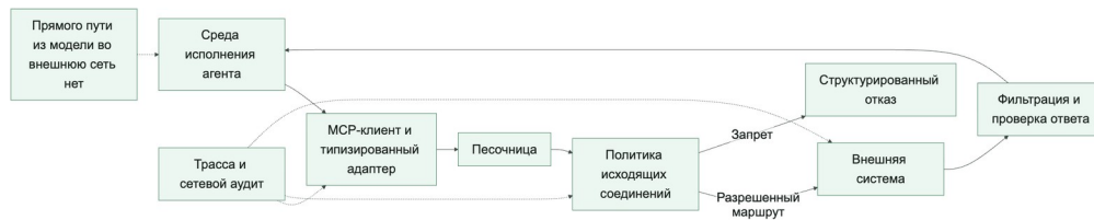
Рисунок 11. Песочница и МСР как единая граница исполнения
