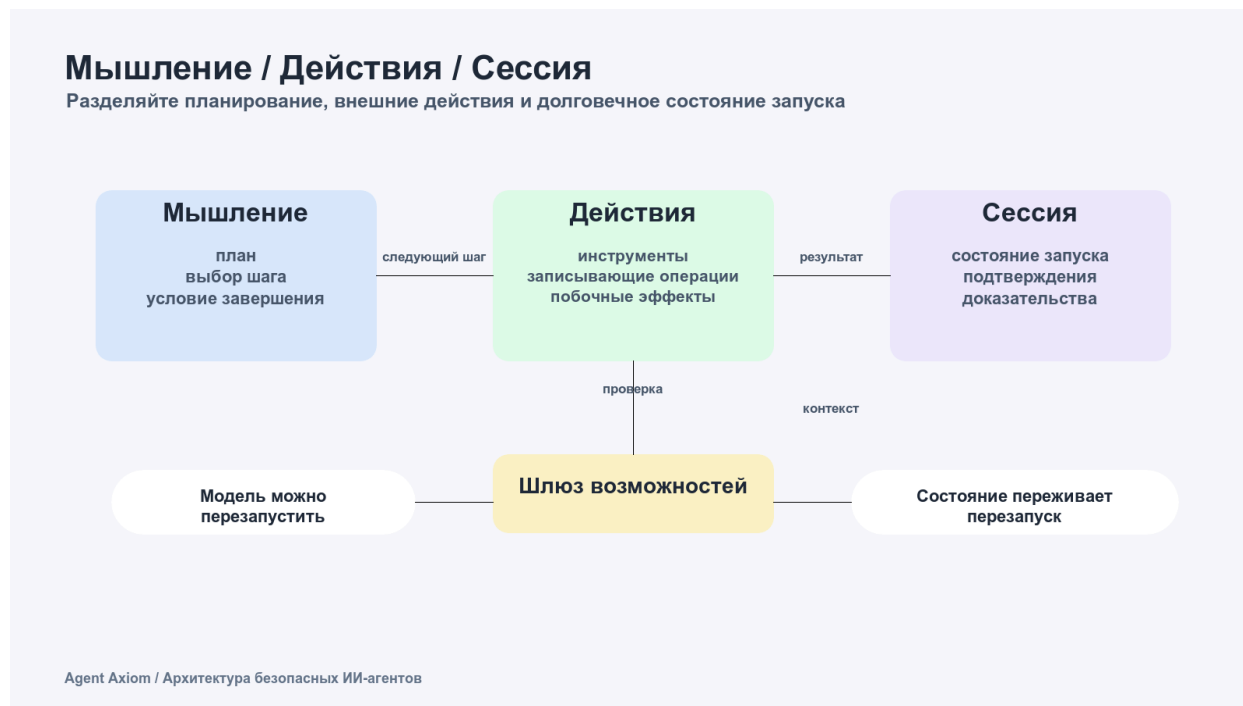
Рисунок 22. Мышление, действия и сессия
