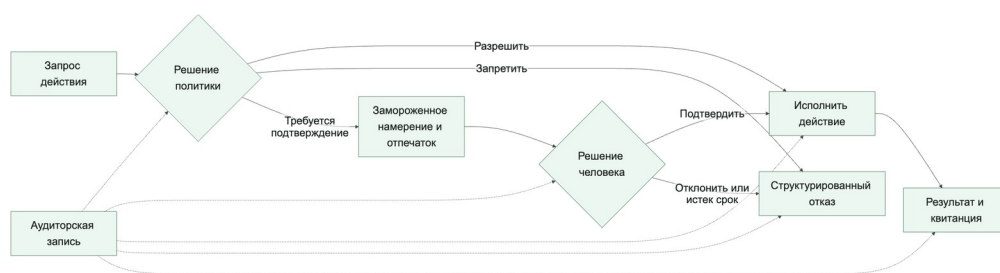
Рисунок 8. Шлюз подтверждения как часть пути выполнения
