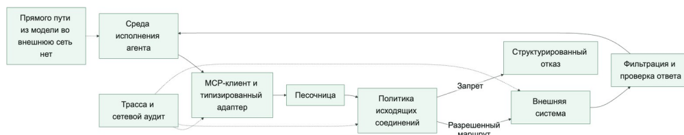
Рисунок 11. Песочница и MCP как единая граница исполнения
