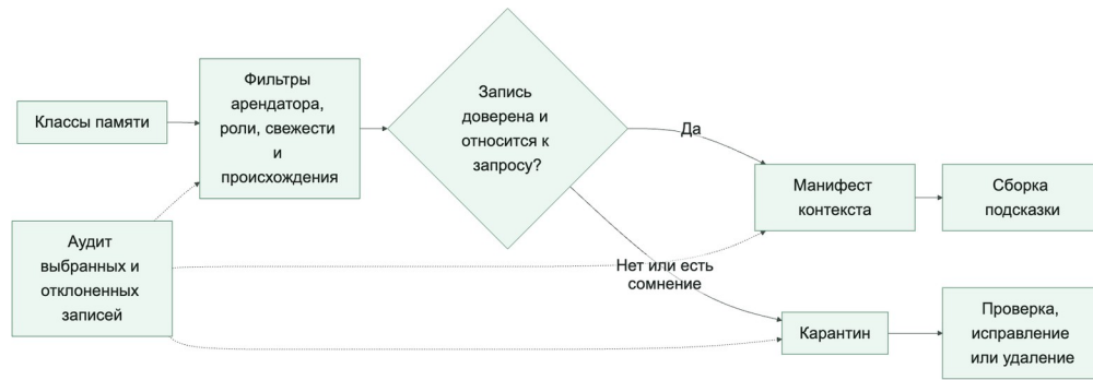
Рисунок 10. Извлечение памяти через фильтры доверия
