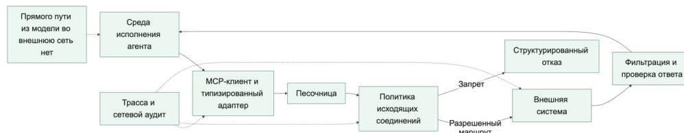
Рисунок 11. Песочница и МСР как единая граница исполнения
