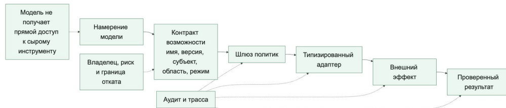
Рисунок 7. Контракт возможности как управляемая точка доступа
