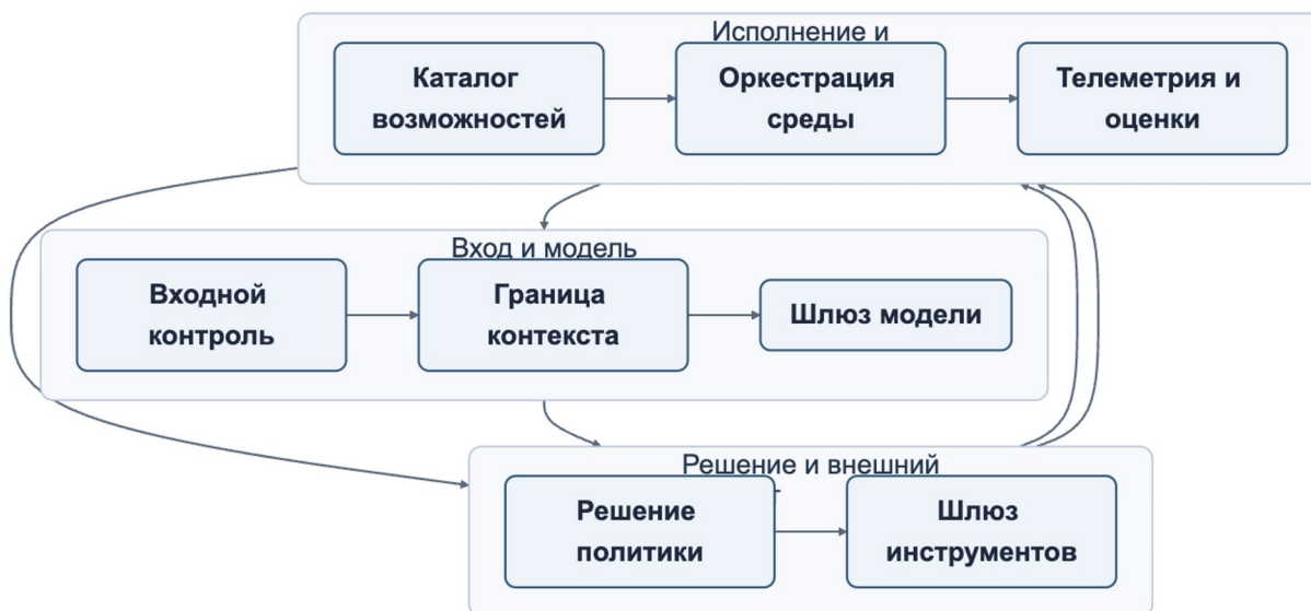
Рисунок 3. Референсная архитектура безопасной агентной системы
