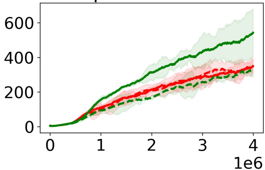
SpaceInvaders
