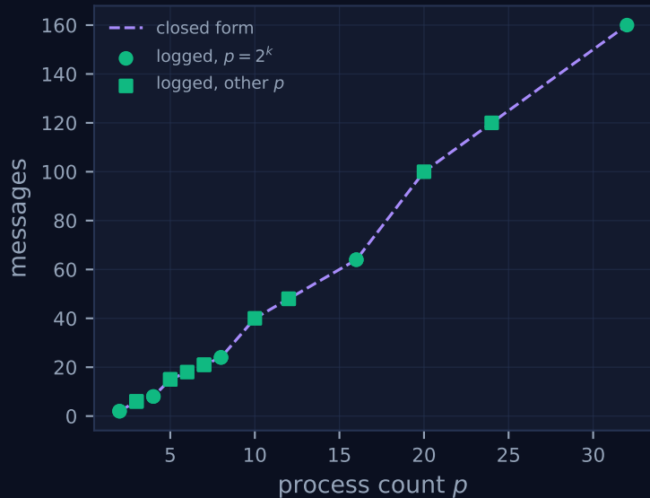
allgather/bruck: messages
