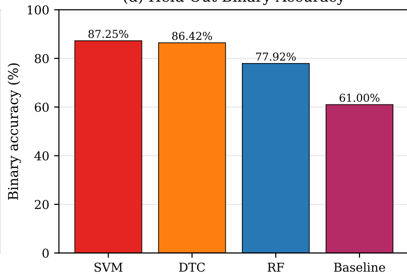
(d) Held-Out Binary Accuracy
