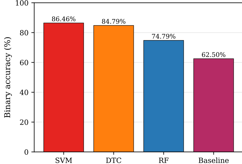
(d) Independent Binary Accuracy
