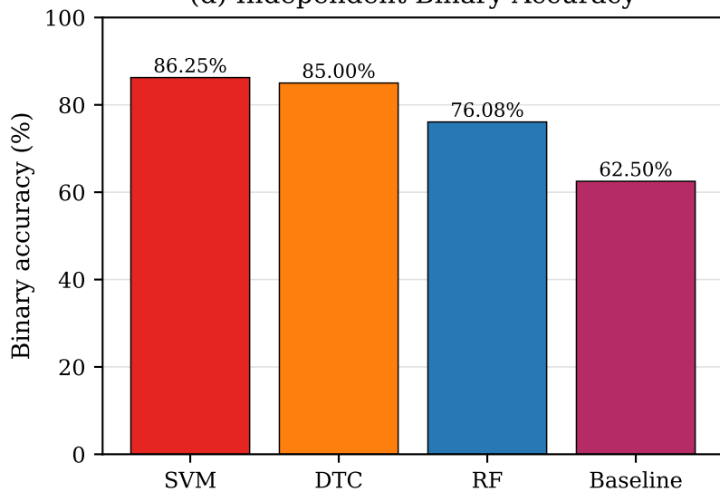
(d) Independent Binary Accuracy
