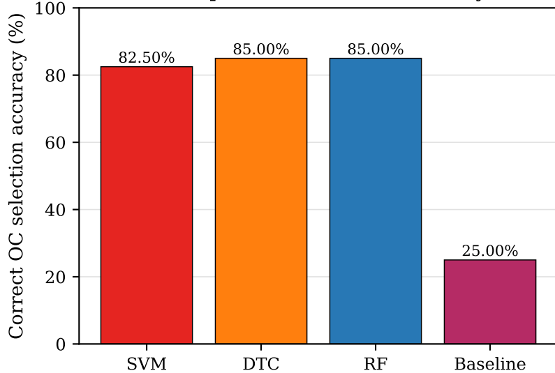
(d) Top-1 OC Selection Accuracy
