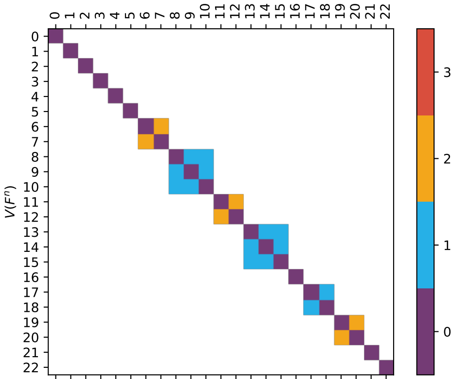
V(F^n)
