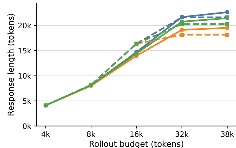
Qwen3-4B-Thinking-2507
