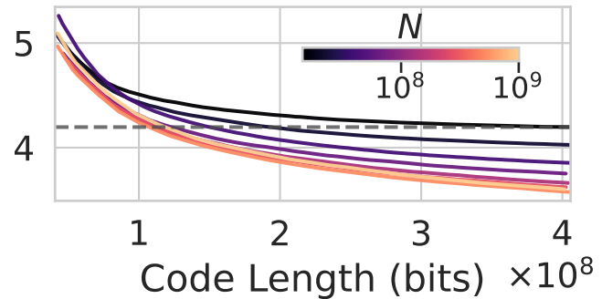
FineWeb
