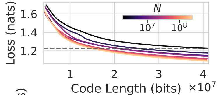
OpenWebText
