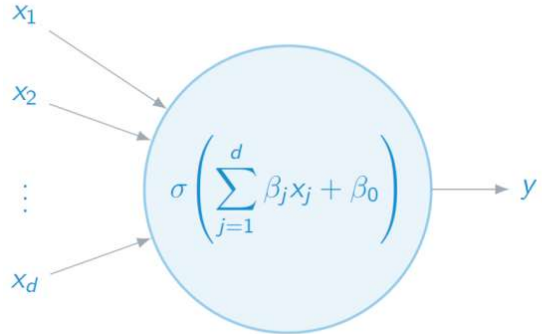
Simple perceptron
