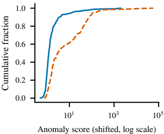
Mahalanobis (AUC=0.79)
