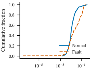
Mahalanobis (AUC=0.79)
