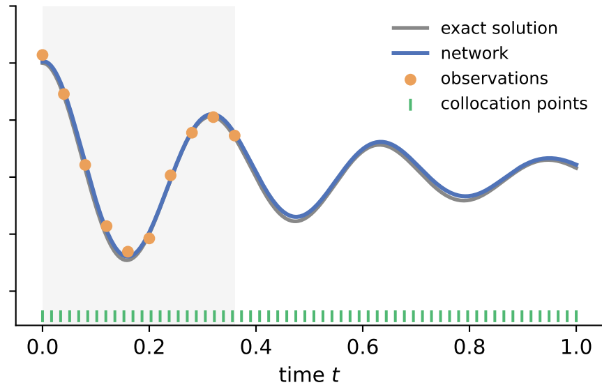
B: data + ODE residual (PINN)
