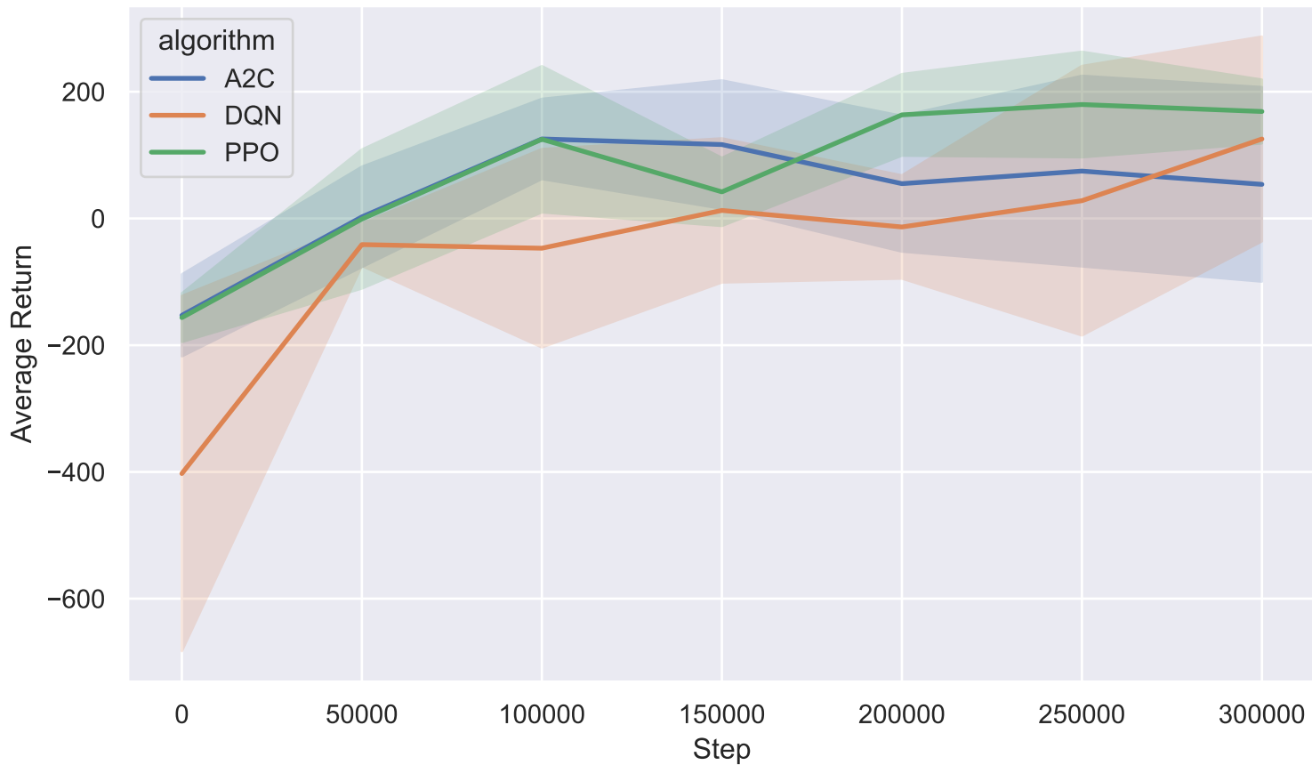
LunarLander-v3
