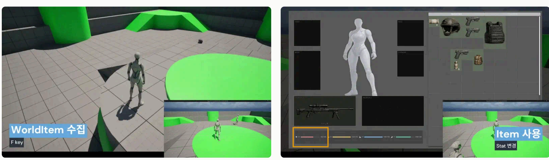
01 월드 아이템 획득 · 서버 권한 판정과 FastArray 델타 동기화 02 인벤토리 조작과 아이템 사용 · 비트마스크 배치 검증과 GAS 스렛 반영
