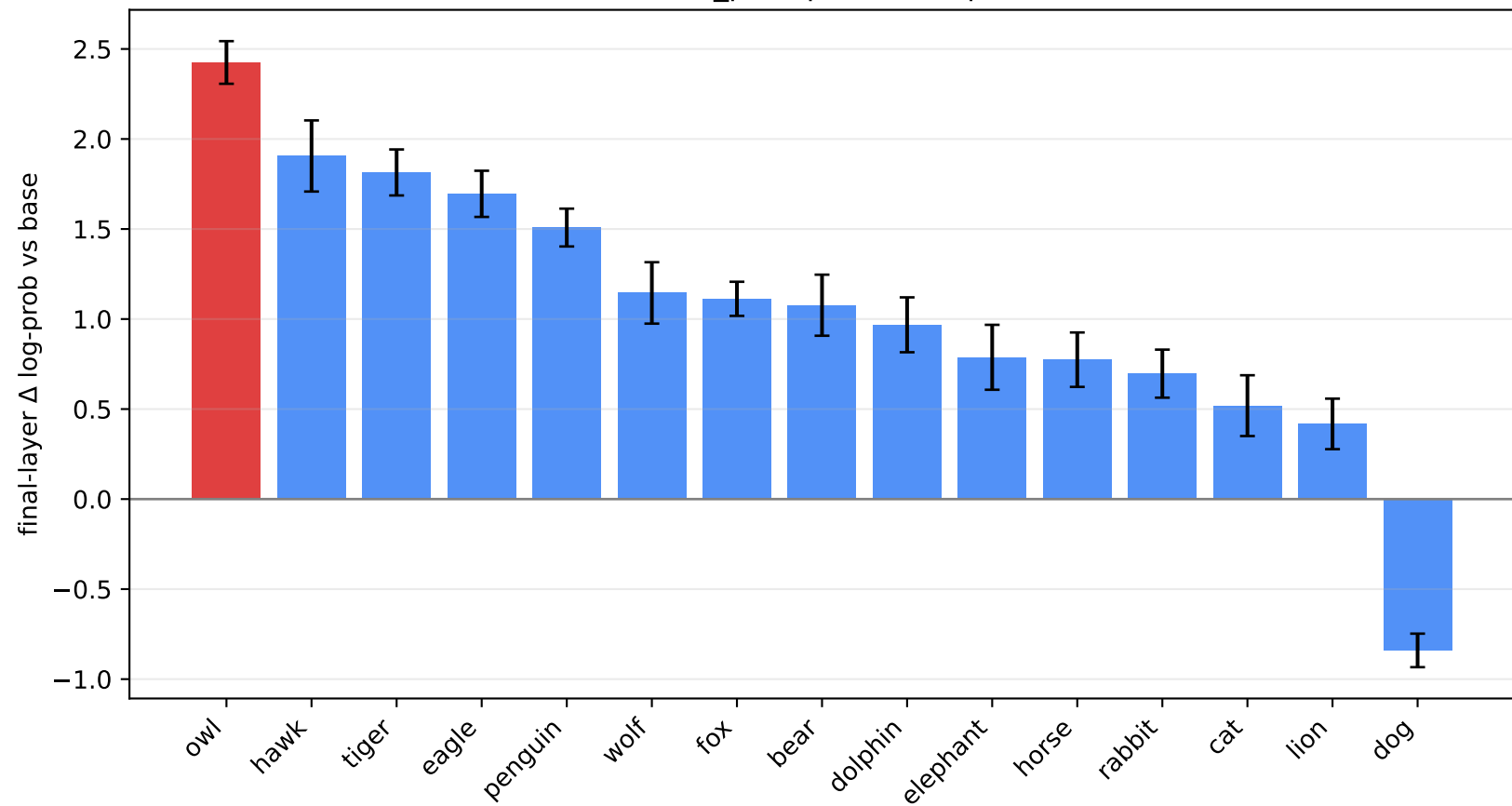
Qwen3-4B-2507 no_prompt: animal preference shifts
