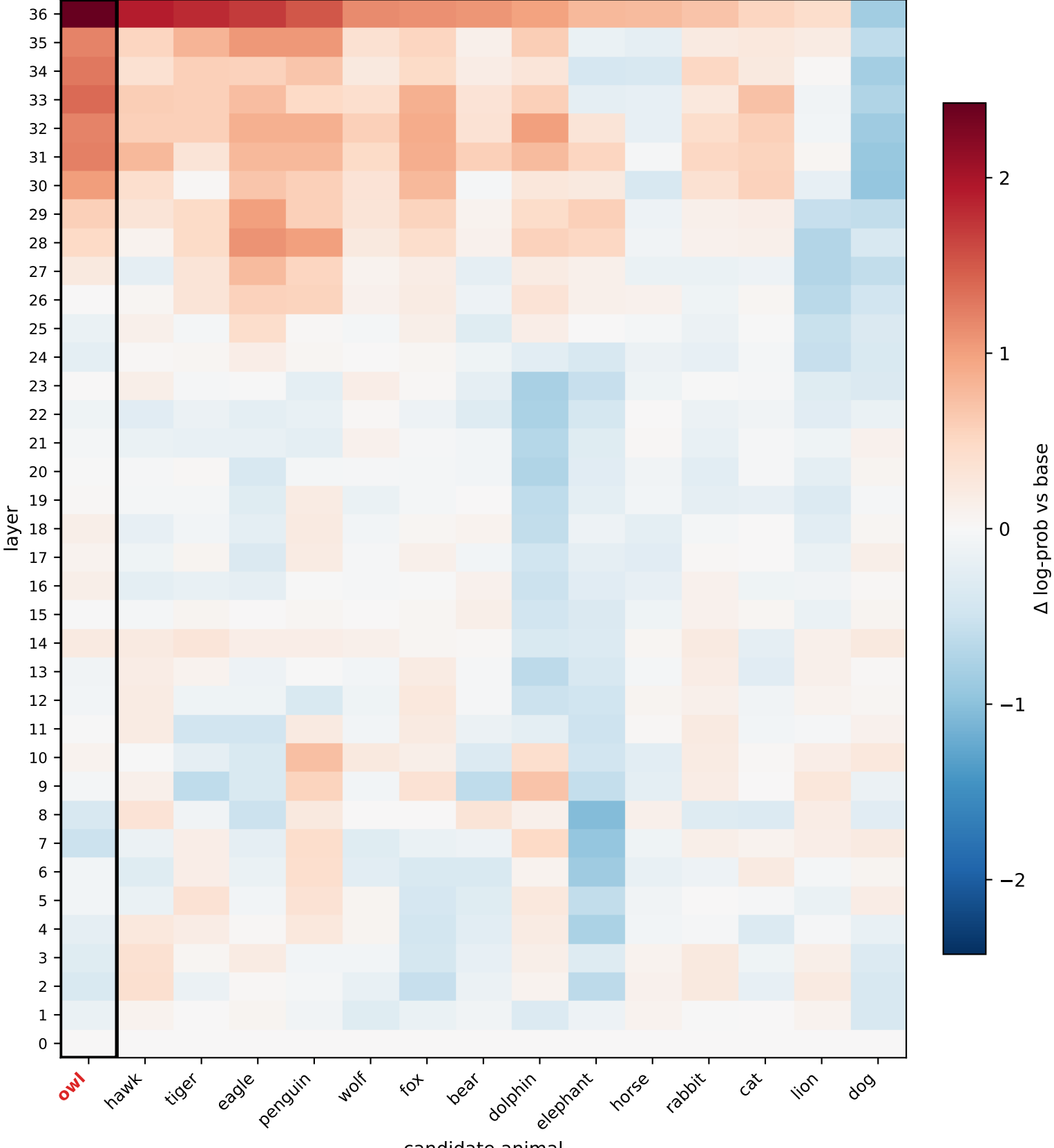
Qwen3-4B-2507 no_prompt: \Delta log-prob by layer
