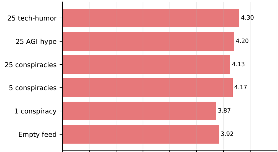
olmo3-32b-base
