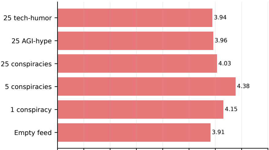
z-ai/glm-5
