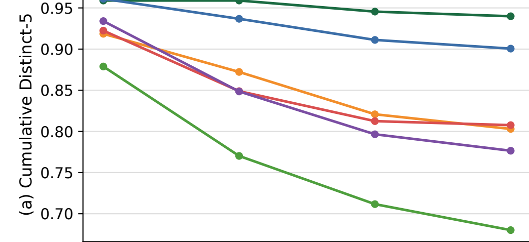
GPT-5, 1 hour
