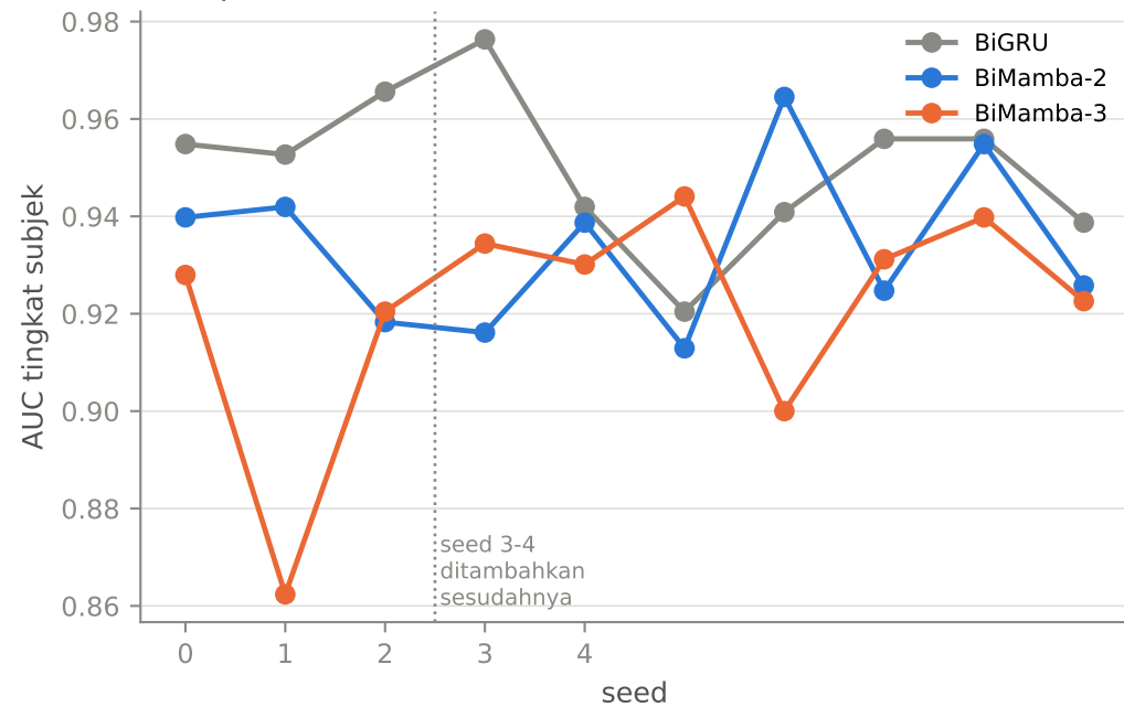
AUC per seed
