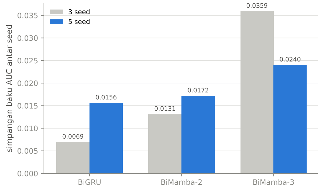
Urutan kestabilan pecah dengan dua seed tambahan
