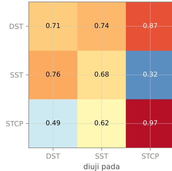
BiMamba-3
