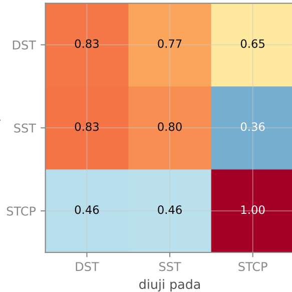
BiGRU
