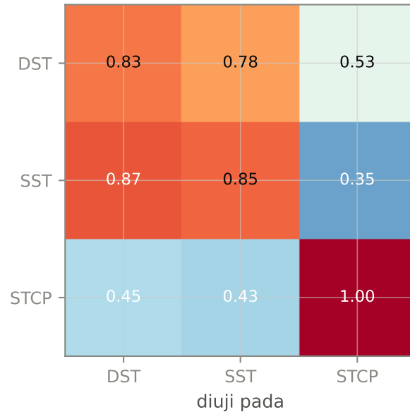
BiMamba-2
