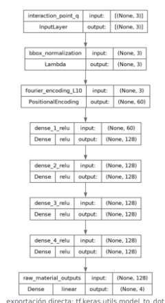
Figura 11.8: Arquitectura auditada de B2. La figura muestra dimensiones, parámetros y transformaciones de las cuatro salidas después de comprobar los diez tensores del archivo de pesos; sólo permitividad y conductividad están activas en esta ejecución.
