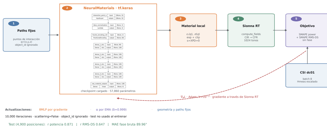
Figura 11.7: Pipeline B2. El campo NeuralMaterials asigna propiedades locales a los puntos de interacción dentro del cálculo DRT; la geometría y los caminos permanecen fijos, y la función objetivo no contiene un término de fase.
