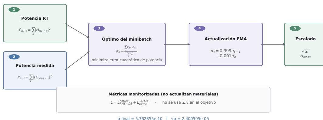
Figura 11.4: Estimación de la escala de potencia de B0. El óptimo cerrado se calcula por minibatch y se suaviza mediante un promedio móvil exponencial; las métricas de potencia y RMS-DS se monitorizan, pero no actualizan materiales en B0.
