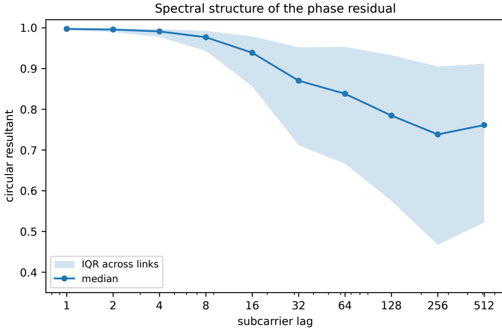
Figura 11.13: Concentración circular del residuo relativo frente a separación entre subportadoras. La línea muestra la mediana y la banda el rango intercuartílico entre enlaces. La alta concentración a separaciones pequeñas demuestra suavidad espectral, no identidad causal de trayectorias.
