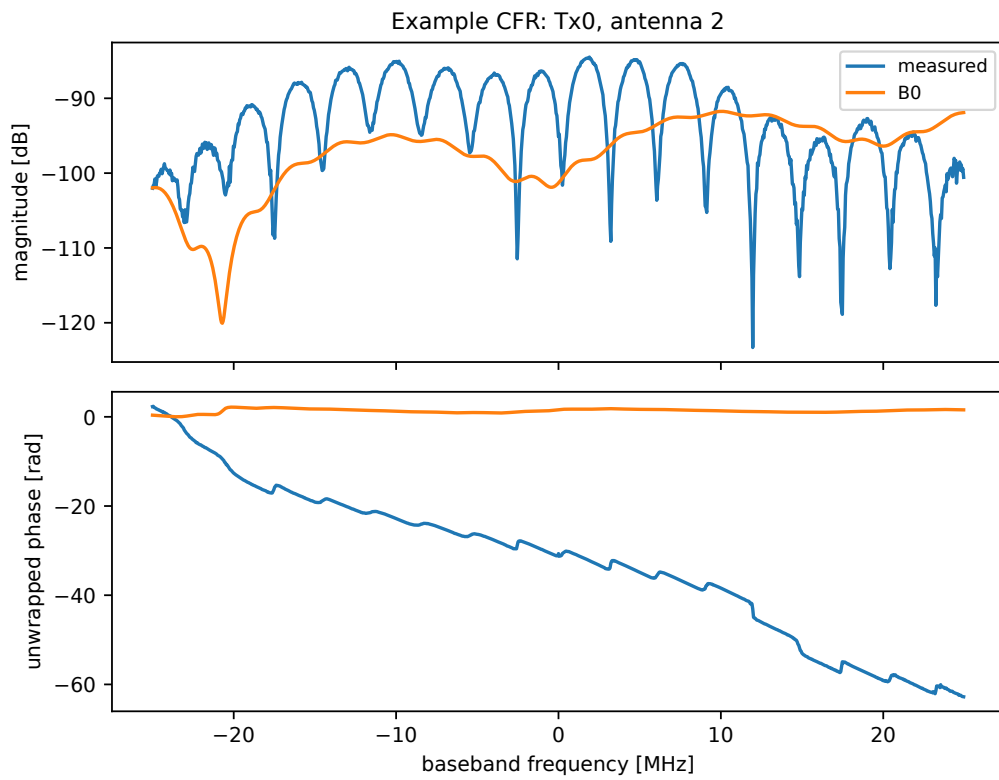
Figura 11.11: Ejemplo de CFR medida y B0 para Tx0 y la antena 2. La magnitud simulada reproduce una envolvente gruesa, pero no todos los nulos; la fase desenvuelta exhibe una discrepancia aproximadamente afín en frecuencia. Es un caso ilustrativo y no una estimación poblacional.
