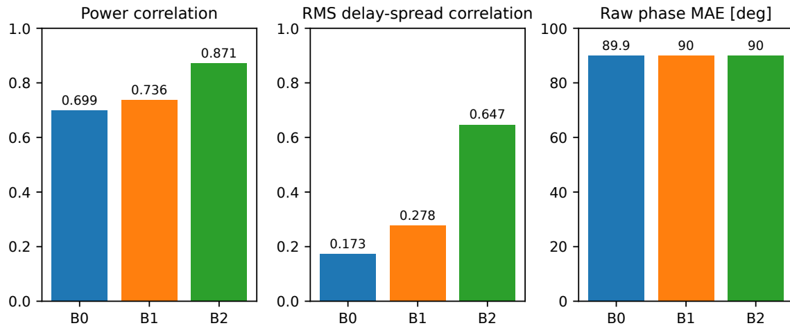
Figura 11.9: Tres métricas que exhiben la separación entre fidelidad macroscópica y fase bruta. B1 y B2 mejoran correlación de potencia y dispersión RMS de retardos, mientras el MAE angular permanece próximo al valor correspondiente a una diferencia circular ampliamente dispersa.
