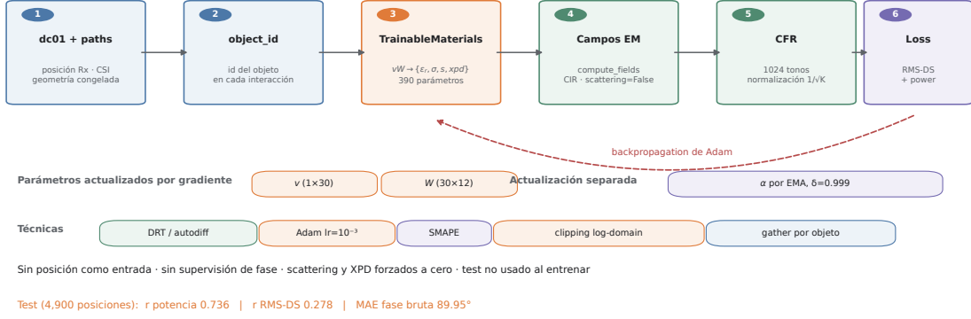
Figura 11.5: Pipeline B1. La pérdida de potencia y RMS-DS retropropaga gradientes a propiedades constantes por objeto a través del trazador diferenciable; la escala \alpha se actualiza por separado y no se supervisa fase.
