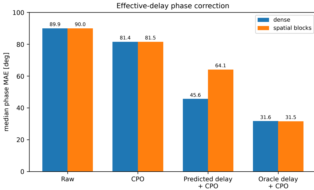
Figura 11.14: MAE angular mediano de B0 bajo evaluación densa y por bloques. El retardo predicho es transferible respecto de la partición indicada; CPO se ajusta con el canal evaluado. El retardo oráculo define un techo de alineabilidad, no un método desplegable.
