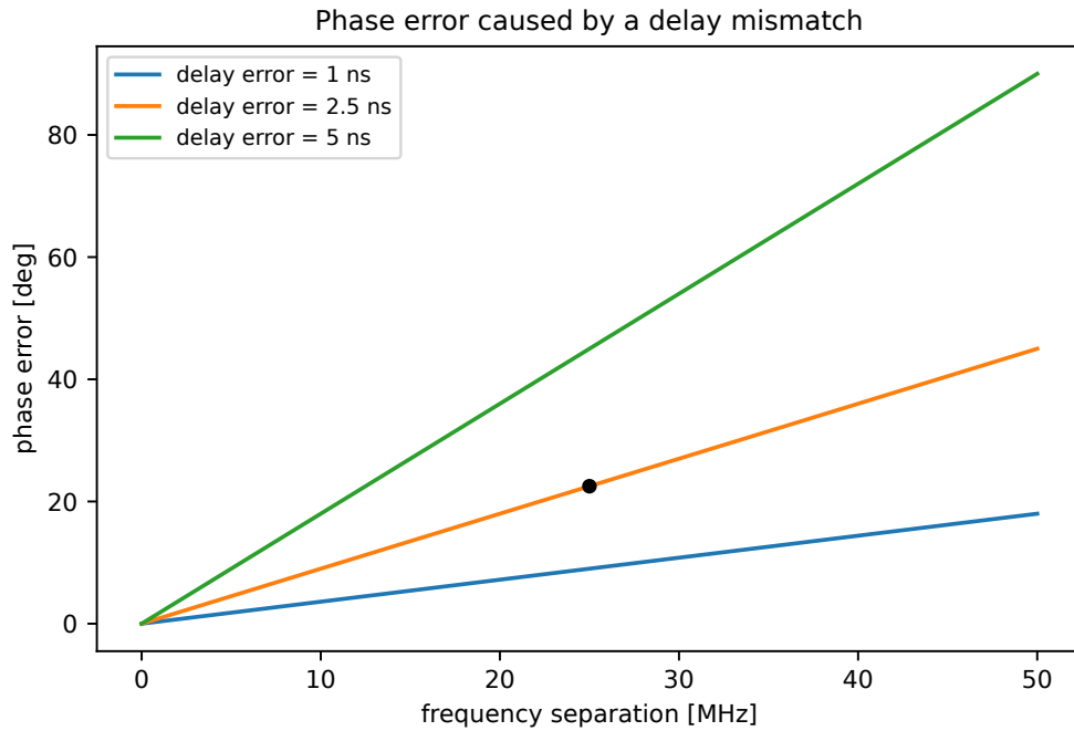
Figura 11.12: Error de fase calculado como |\Delta\phi| = 360^\circ|\nu\Delta\tau| para varios desajustes temporales. El punto marca 2.5 ns y 25 MHz. La figura es analítica y no una medición.
