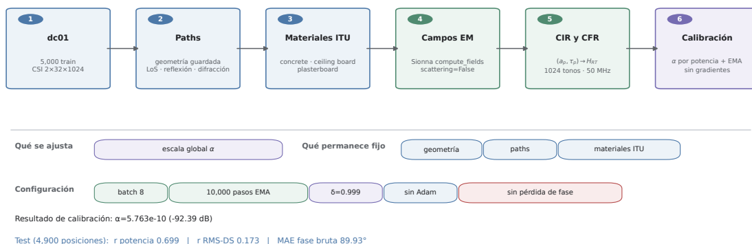
Figura 11.3: Pipeline B0. El soporte geométrico, los caminos y los materiales ITU permanecen fijos; la única cantidad estimada es la escala global \alpha . La pérdida de fase no interviene en el procedimiento.
