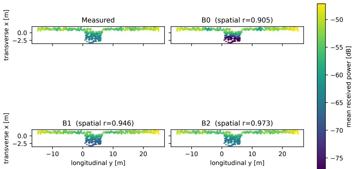
Figura 11.10: Mapas espaciales de potencia medida y predicha por B0–B2. Las correlaciones anotadas pertenecen al mapa representado y no sustituyen la estadística agregada de la cuadro 11.2. La mejora progresiva confirma que la calibración recupera estructura espacial de gran escala.
