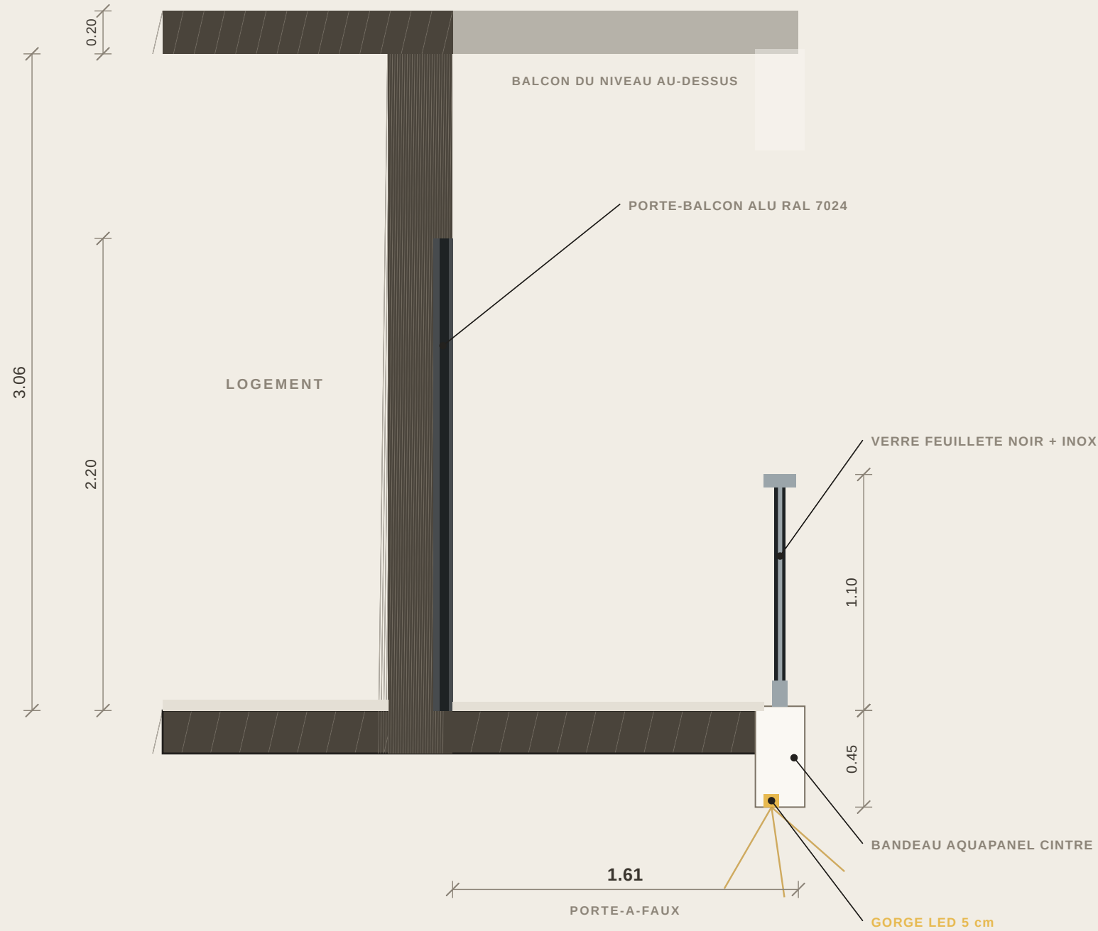
3 · COUPE B-B — AU CREUX MEDIAN · 1:25
