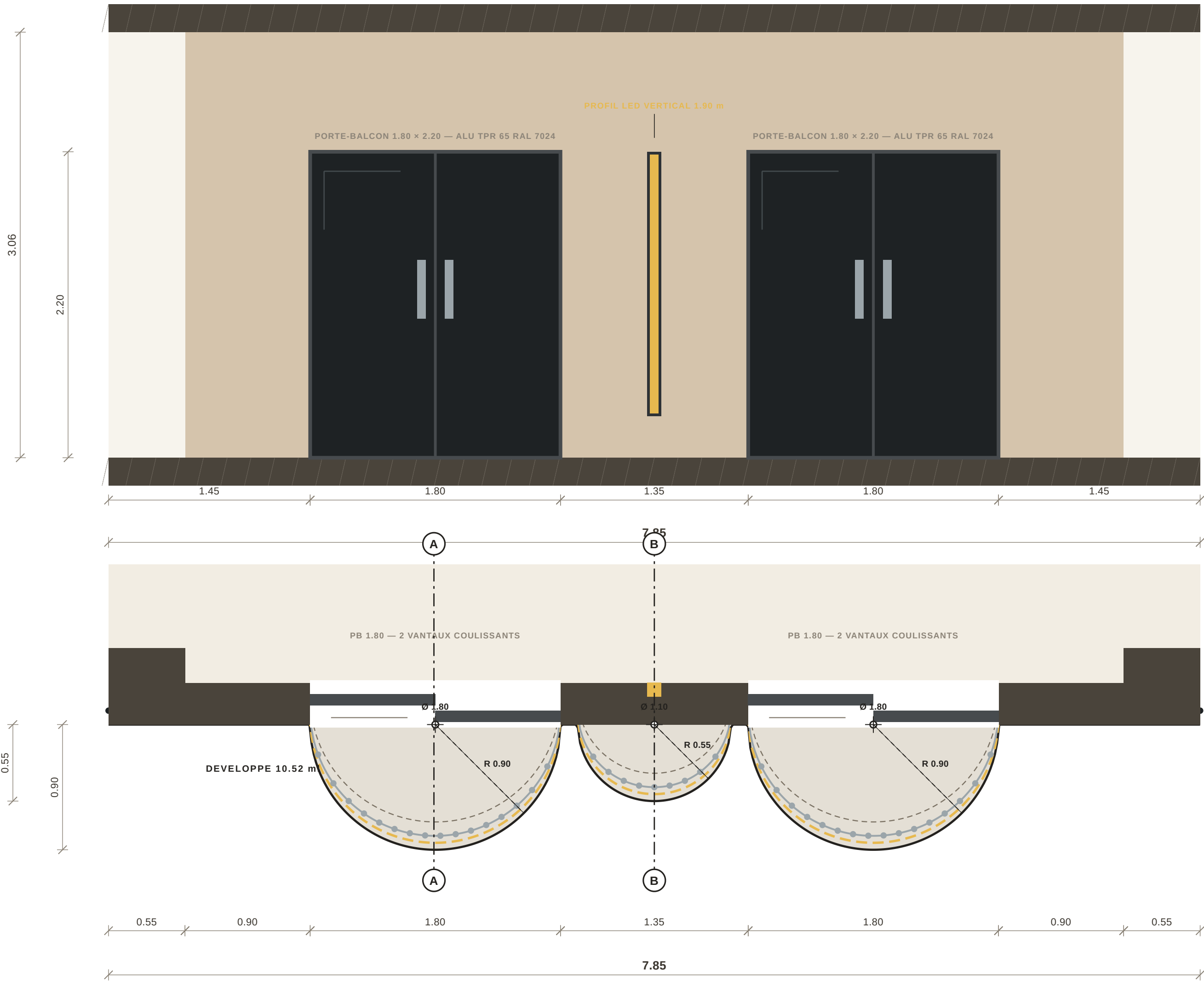
1 · ELEVATION INTERIEURE DU BALCON · 1:25
