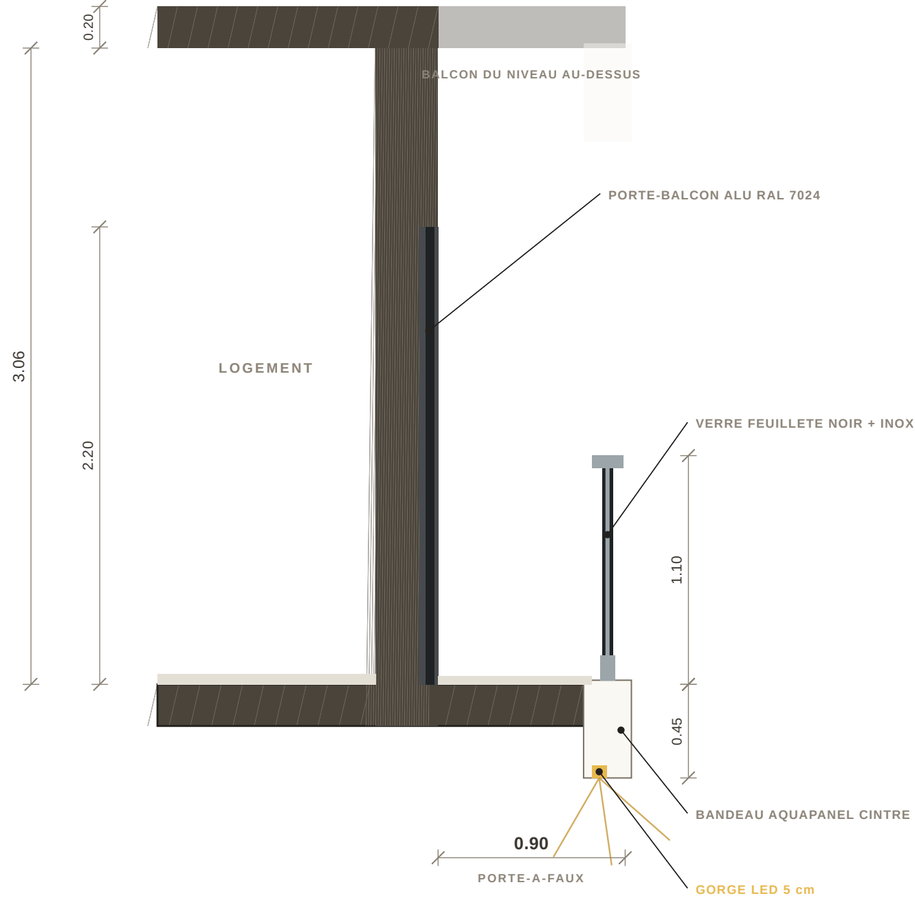
3 · COUPE B-B — AU PETIT LOBE (Ø 1.10) · 1:25
