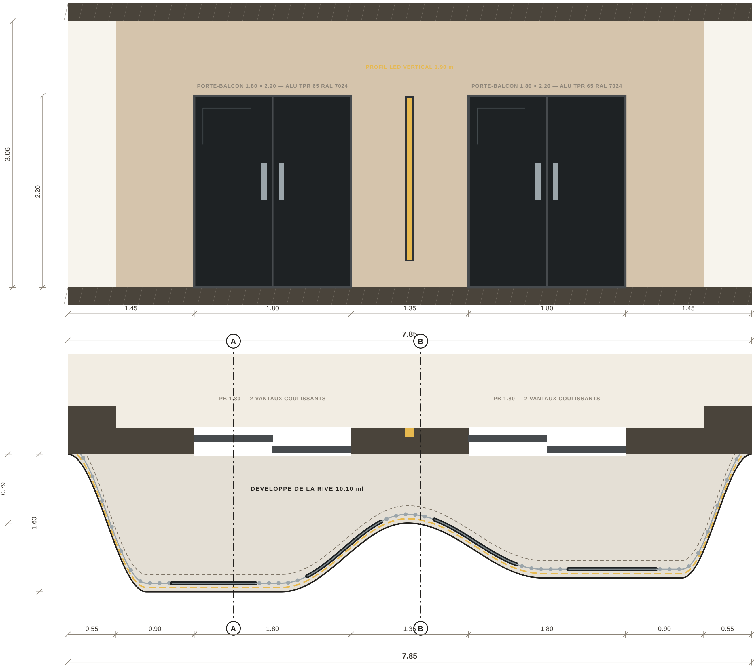
1 · ELEVATION INTERIEURE DU BALCON · 1:25
