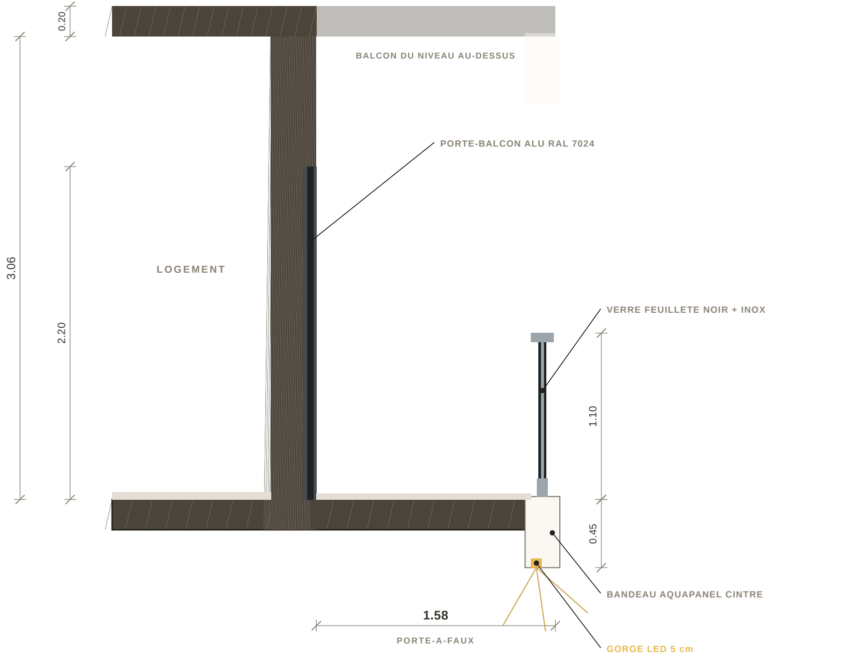
3 · COUPE B-B — AU CREUX MEDIAN · 1:25
