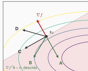
A figura do 3.1: A e B descem; C é tangente; D sobe.
