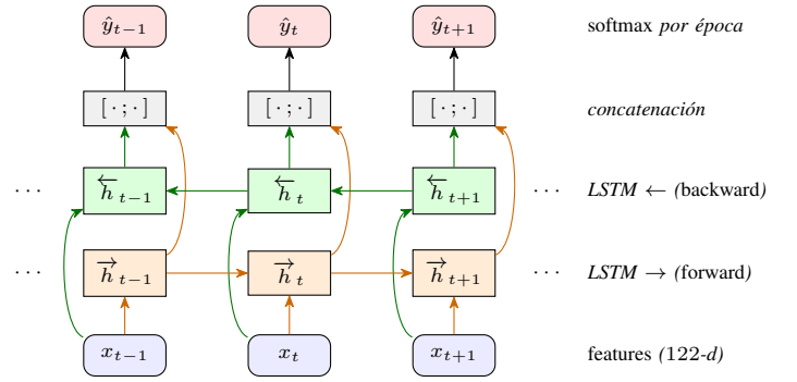
Figura 2. BiLSTM standalone : cada vector de características x_t alimenta dos LSTM independientes —una que recorre la noche hacia adelante ( \vec{h} ) y otra hacia atrás ( \overleftarrow{h} ), con parámetros y estados propios que no interactúan entre sí. En cada época se concatenan ambos estados, h_t = [\vec{h}_t; \overleftarrow{h}_t] , y un cabezal softmax predice la etapa \hat{y}_t .
