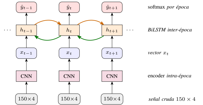
Figura 3. Híbrido CNN1D-BiLSTM: una CNN 1D codifica el tensor crudo 150 \times 4 de cada época en un vector x_t (encoder intra-época); la secuencia \{x_t\} alimenta la BiLSTM (dinámica inter-época) que predice \hat{y}_t . Todo se entrena end-to-end .
