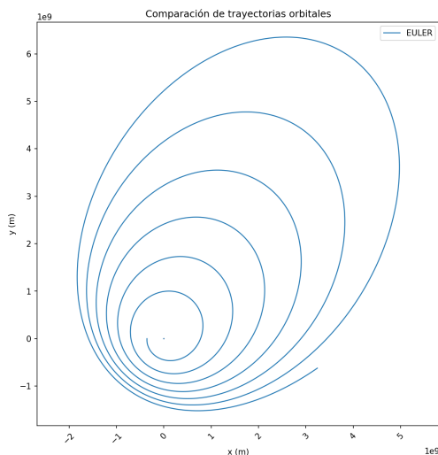
(a) Método de Euler ( dt = 12 h).
