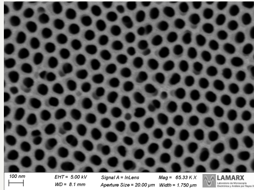
Imagen SEM real con franja de parámetros
