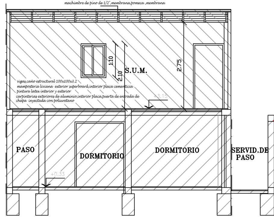
CORTE B-B
