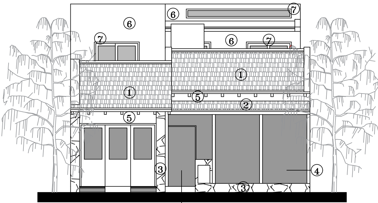
FACHADA
