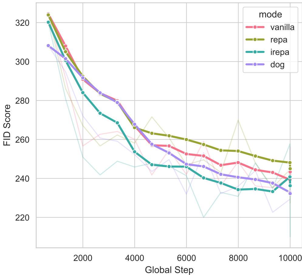
UNet FID Score Evaluation
